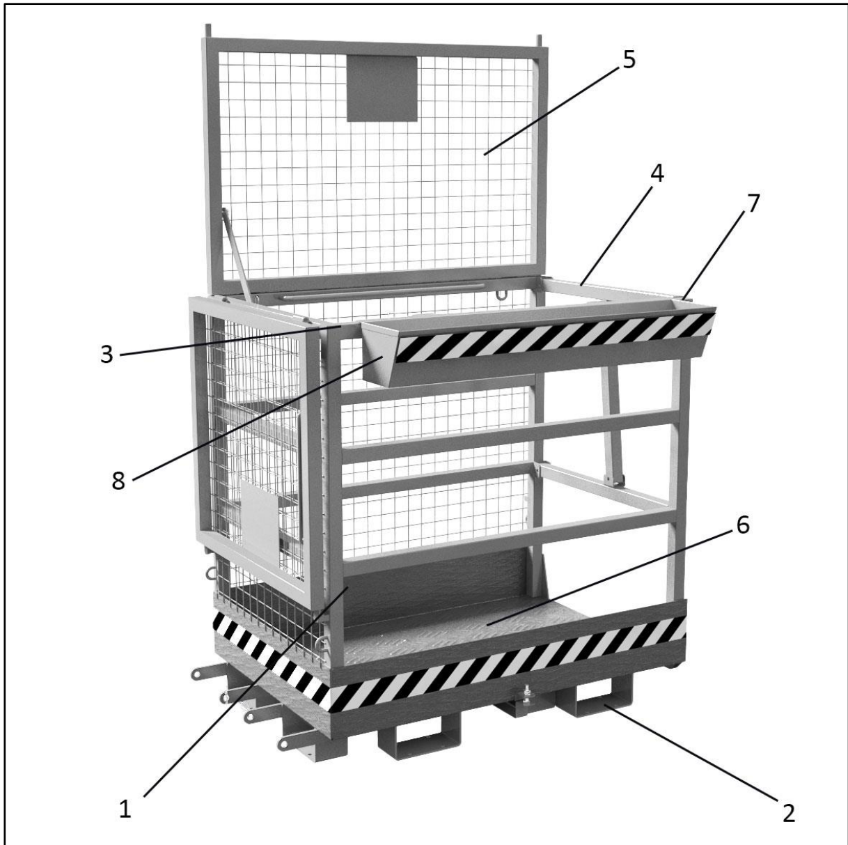
Obr. 2: Obslužná plošina na vidlice
